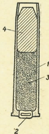
Рис. 25. Боевой патрон в разрезанном виде: 1 — гильза; 2 — капсюль; 3 — заряд; 4 — пуля
