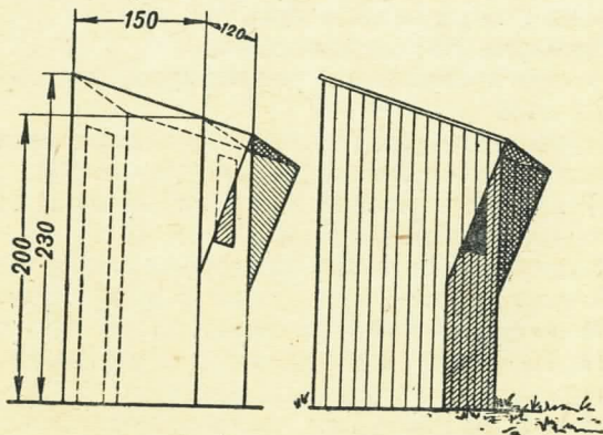
Рис. 42. Будка (размеры в см)
