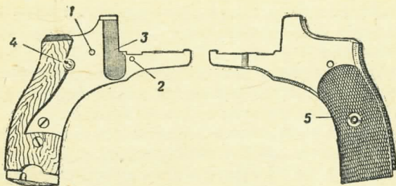
Рис. 9. Боковая крышка:
