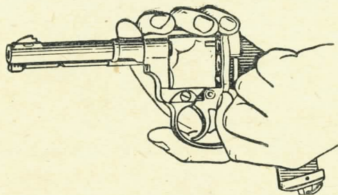
Рис. 34. Как вынуть собачку
