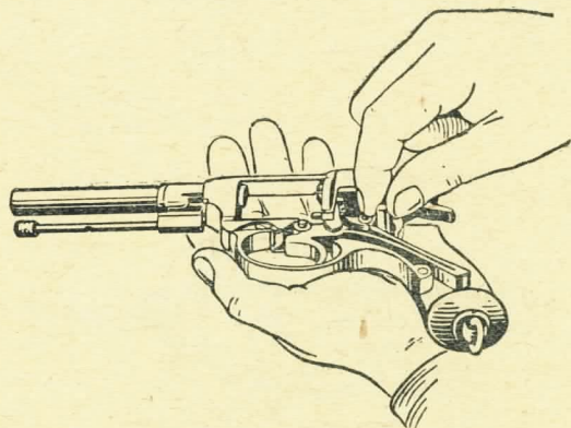
Рис. 32. Как ввинтить соединительный винт
