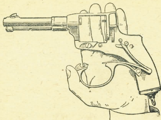
Рис. 38. Как освободить боевую пружину
